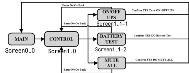
Экран 1.0. Дерево раздела управления
